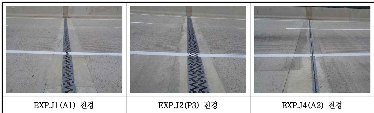
【사진 20.3.16】 신축이음장치 전경
