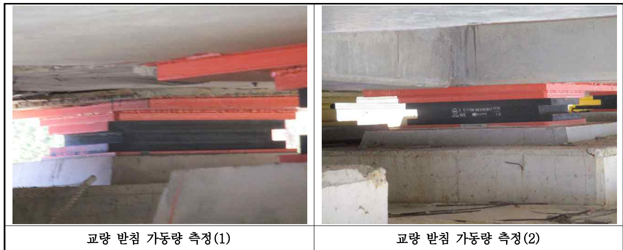
【사진 20.3.38】 교량받침 이동량 측정
