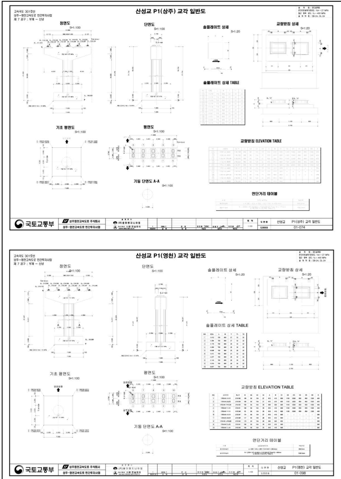
【그림 20.1.7】 교각 일반도
