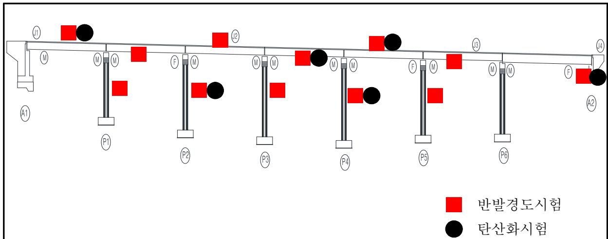
【그림 1.4.2】 영천방향 콘크리트 내구성조사 위치도
