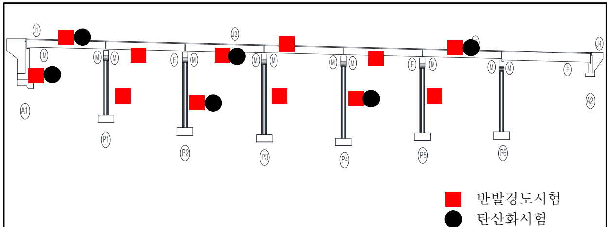
【그림 1.4.1】 상주방향 콘크리트 내구성조사 위치도
